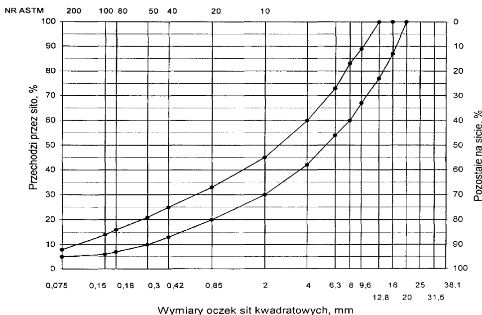
Rys. 1. Krzywe graniczne uziarnienia mieszanki mineralnej BA od 0 do 16 mm do warstwy wyrównawczej nawierzchni drogi o obciążeniu ruchem KR6.
