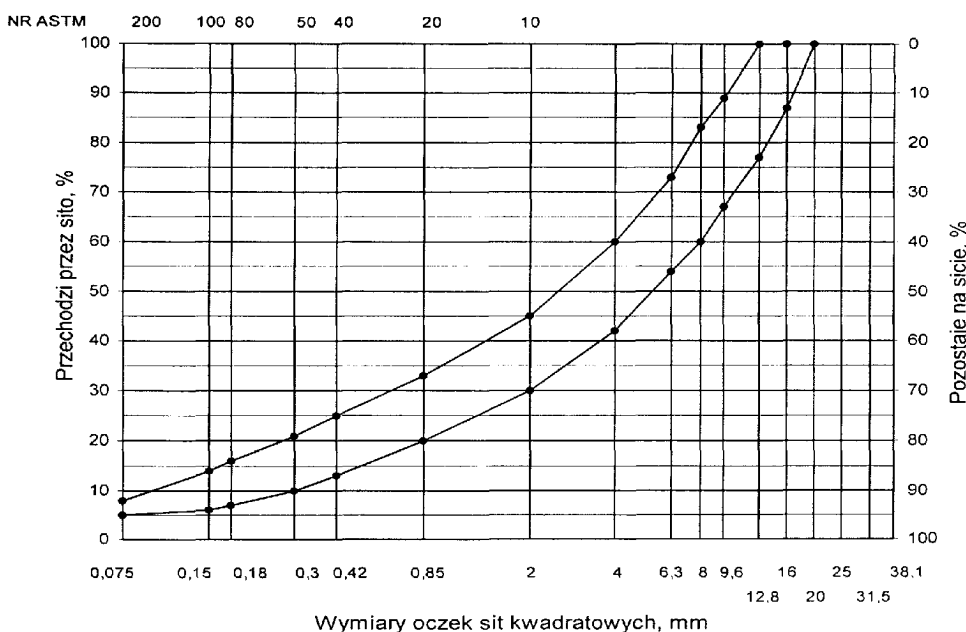
Rys. 1. Krzywe graniczne uziarnienia mieszanki mineralnej BA od 0 do 16 mm do warstwy wyrównawczej nawierzchni drogi o obciążeniu ruchem KR6.
