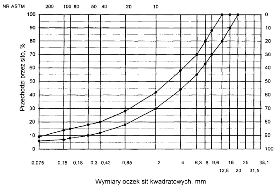
Rys. 1. Krzywe graniczne uziarnienia mieszanki mineralnej BA od 0 do 16 mm do warstwy ścieralnej nawierzchni drogi o obciążeniu ruchu KR6
