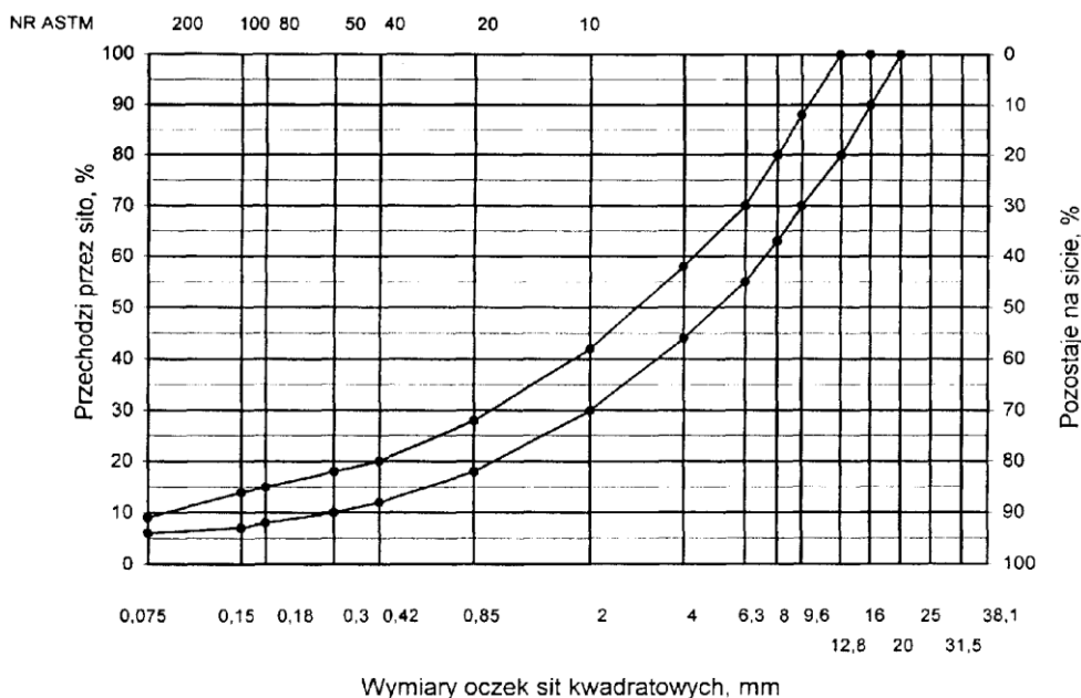
Rys. 1. Krzywe graniczne uziarnienia mieszanki mineralnej BA od 0 do 16 mm do warstwy ścieralnej nawierzchni drogi o obciążeniu ruchem KR6
